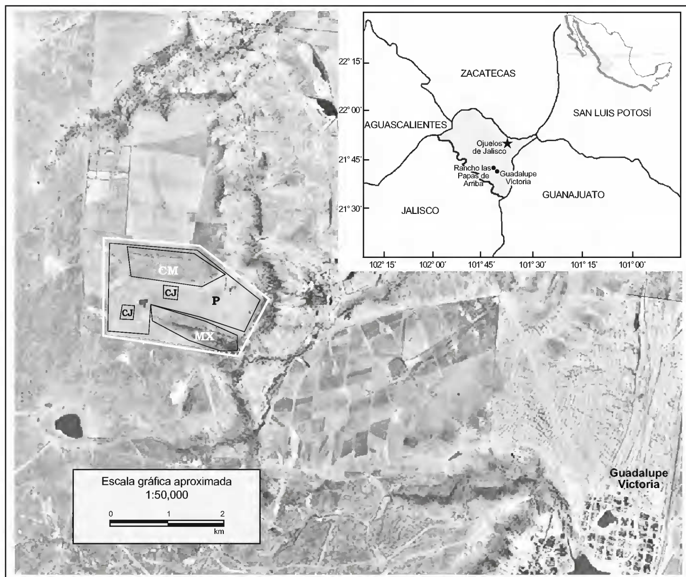
Fig. 1. Ubicación del área de estudio y los sitios de recolecta en el rancho Las Papas de Arriba, municipio de Ojuelos de Jalisco, Jalisco, México: matorral xerófilo crasicauale (MX), pastizal (P), cultivo maduro de nopal tunero (CM), cultivo joven de nopal tunero (CJ). (Fotografía aérea INEGI, 1991)
